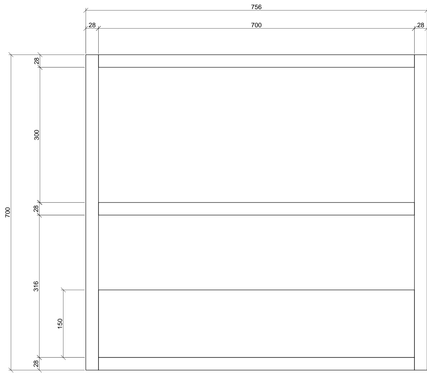
ALZADO
