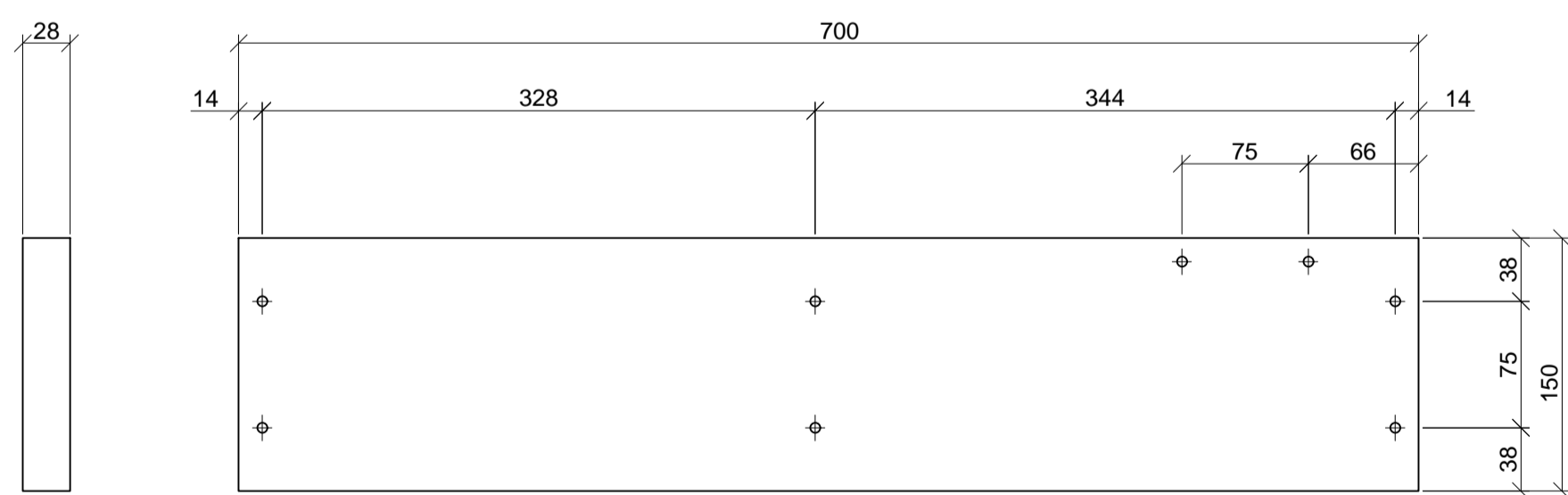
P1 A: DOS TABLAS LATERALES CON AGUJEROS EN LOS QUE IRÁN LOS TORNILLOS DE LAS DEMÁS TABLAS.
