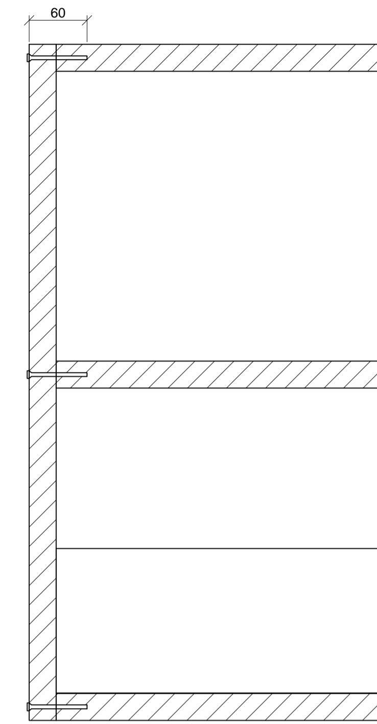
SECCIÓN BB'
